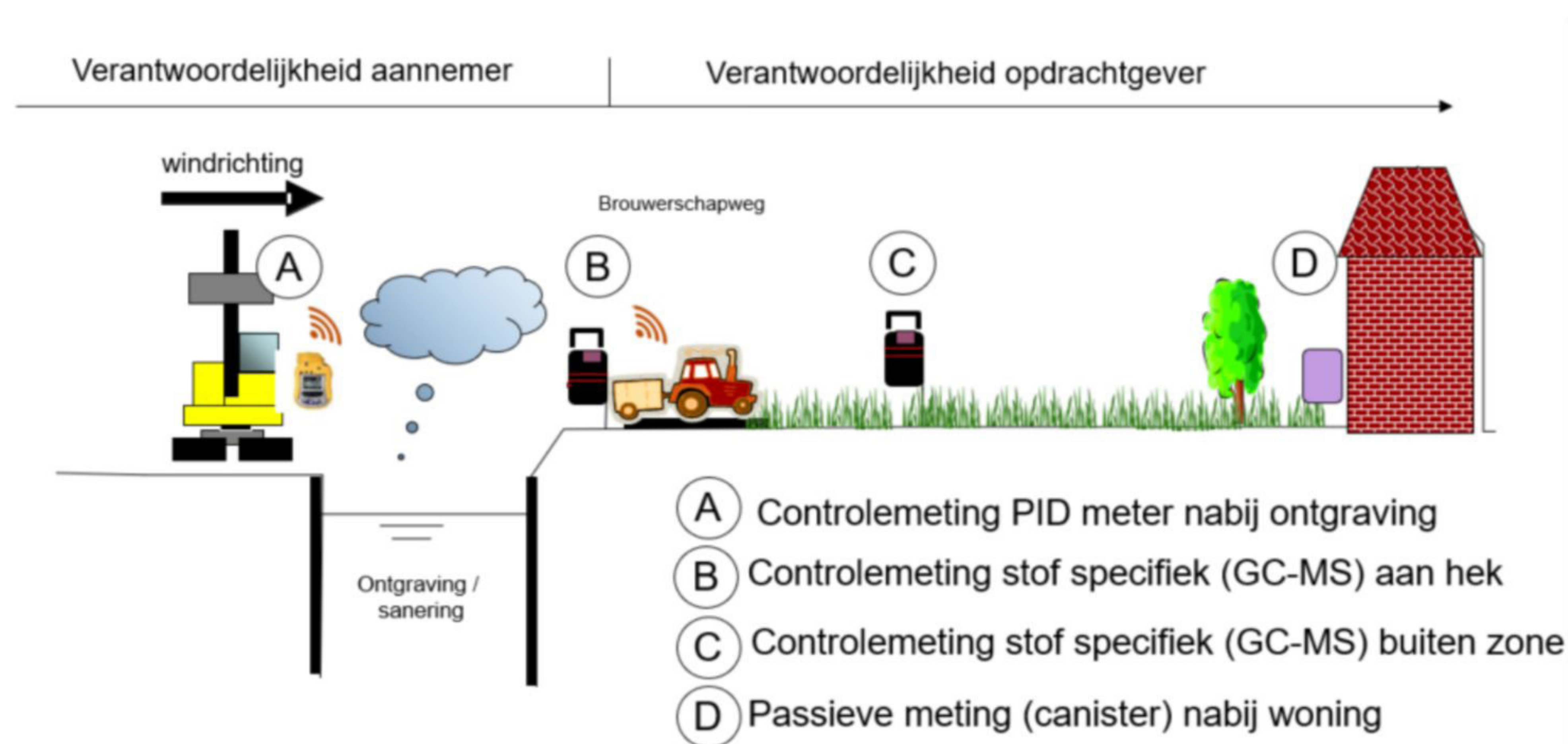
Figuur 5.2 Meetstrategie
