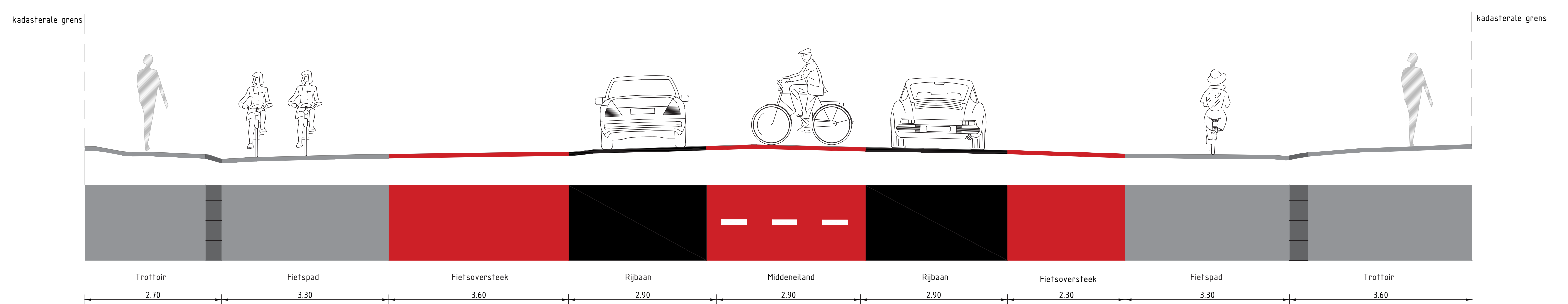
Profiel (DP03) t.h.v. oversteek Rijksstraatweg naar entree Campus Esserberg 1:50
