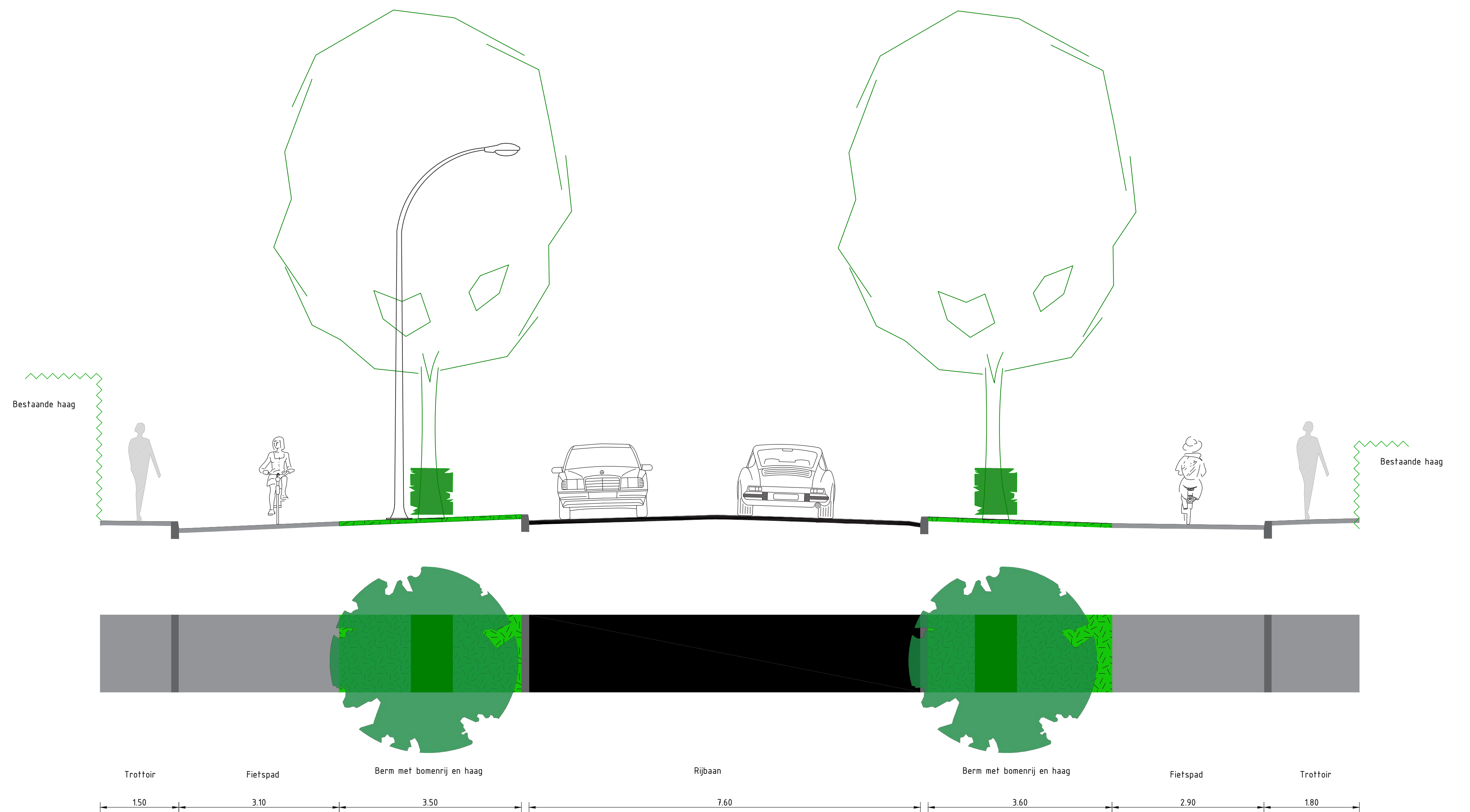
Profiel (DP02) Rijksstraatweg tussen ingang Be Quick en ingang naar Campus Esserberg 1:50
