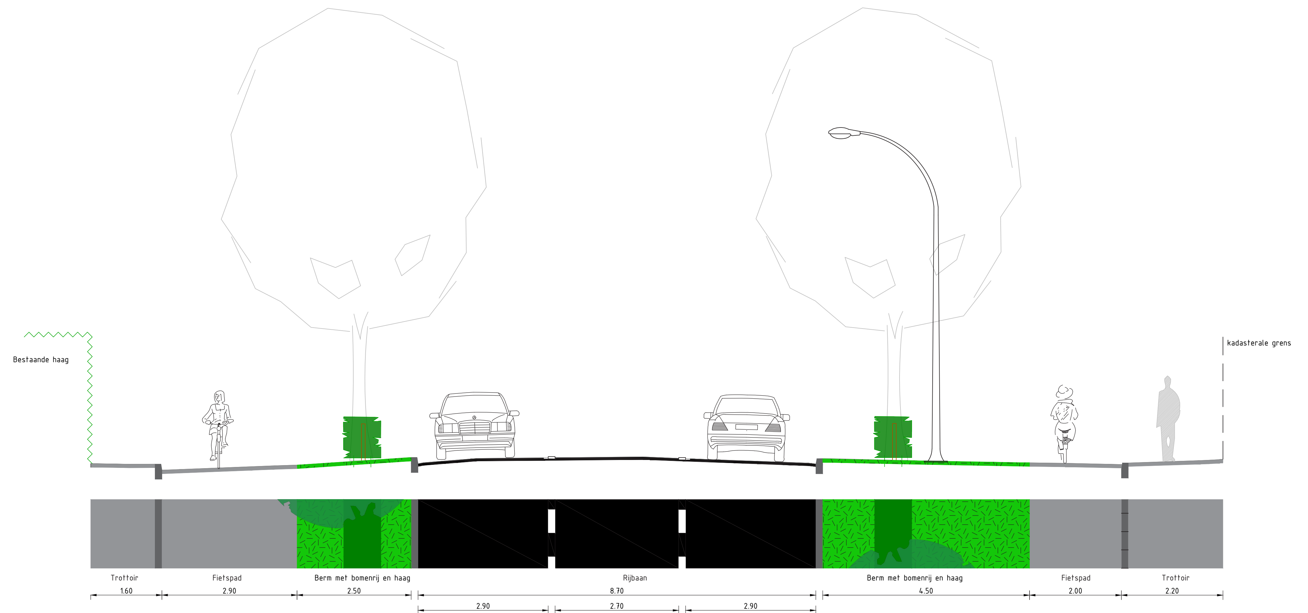
Profiel (DP01) Rijksstraatweg t.h.v. ingang naar Be Quick 1:50
