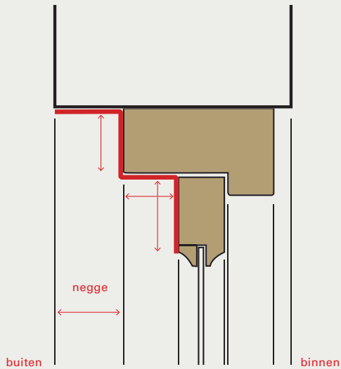
OORSPRONKELIJKE SITUATIE
