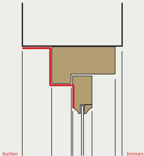
OORSPRONKELIJKE SITUATIE
