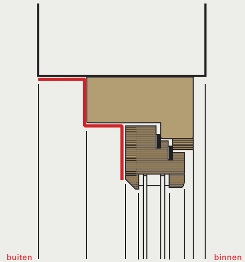
NIEUWE SITUATIE
