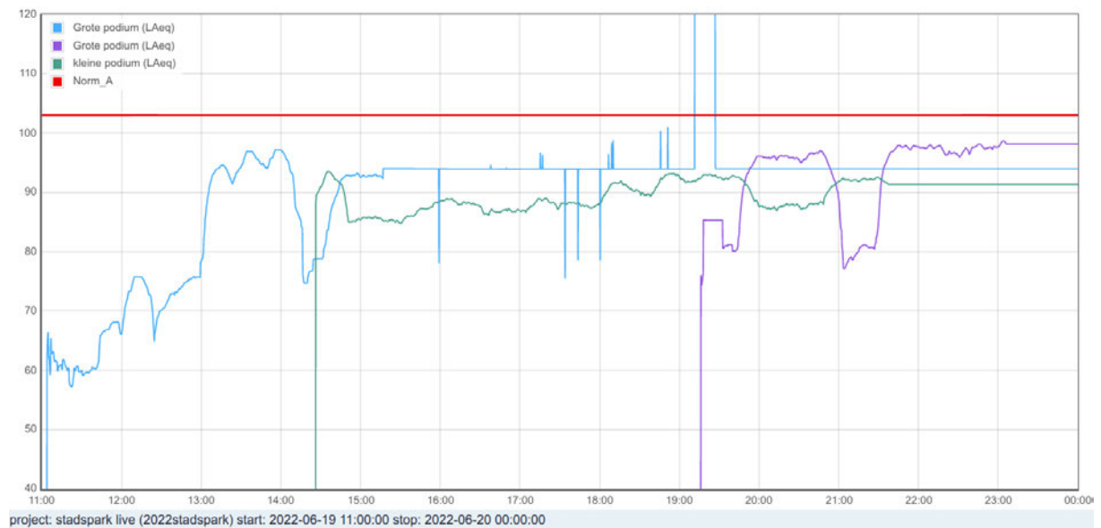
Figuur 12: Meetresultaten foh, dB(A)
