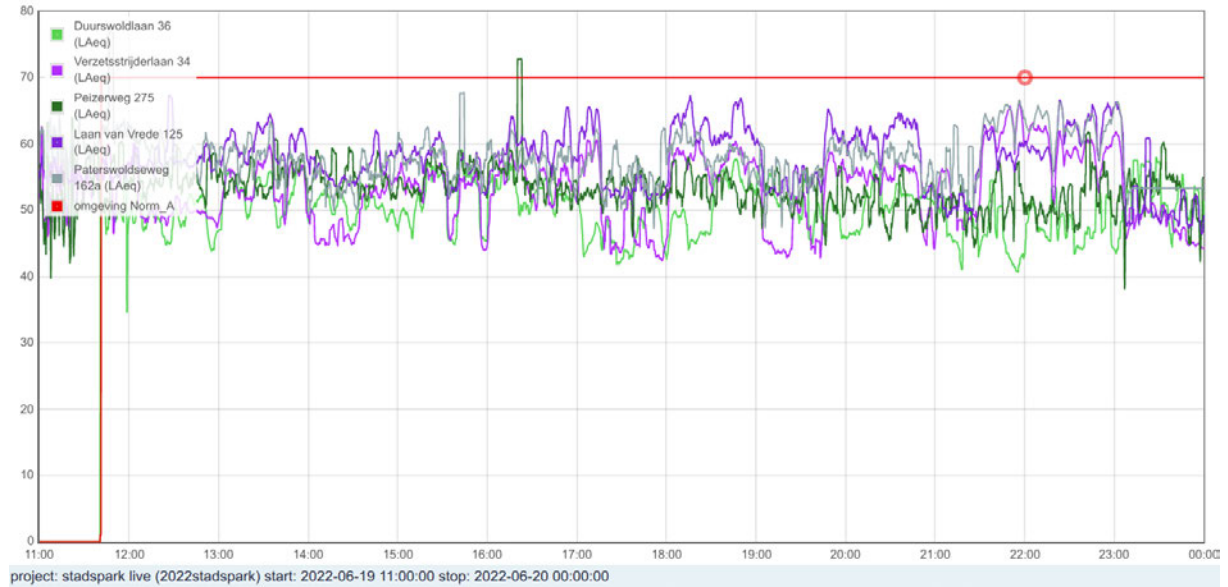
Figuur 8: Meetresultaten omgeving, dB(A)
