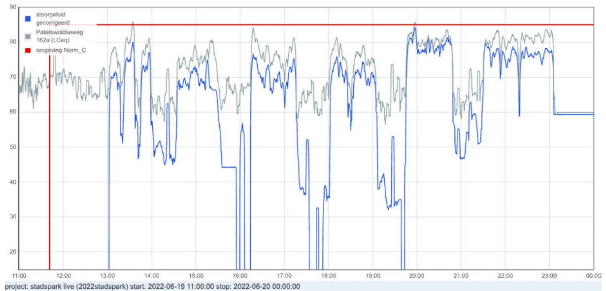
Figuur 11: : Meetresultaten Paterwoldseweg, dB(C), stoorgeluid gecorrigeerd
