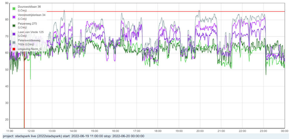
Figuur 10: Meetresultaten omgeving, dB(C)
