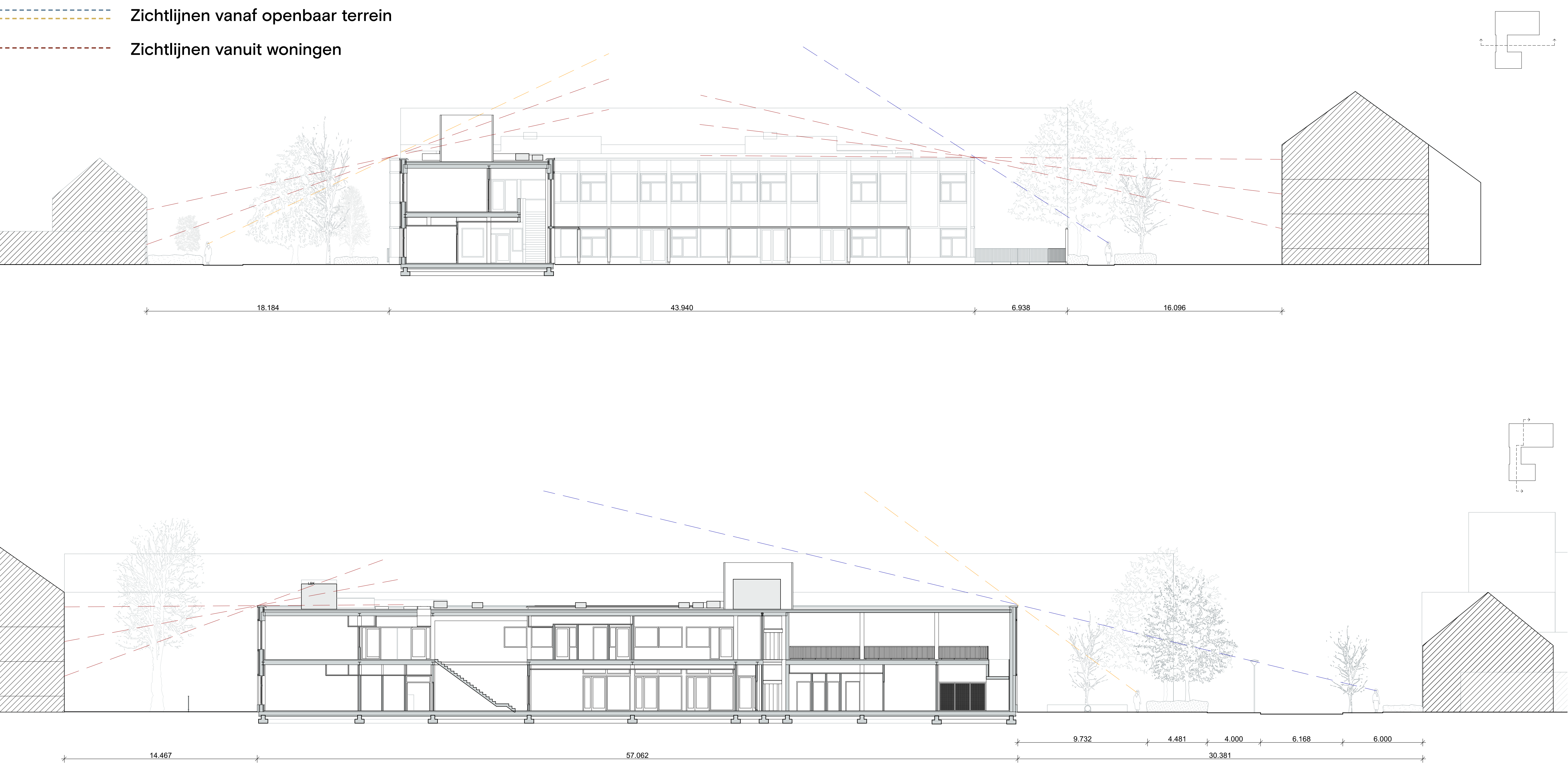
Doorsnedes 1:150
