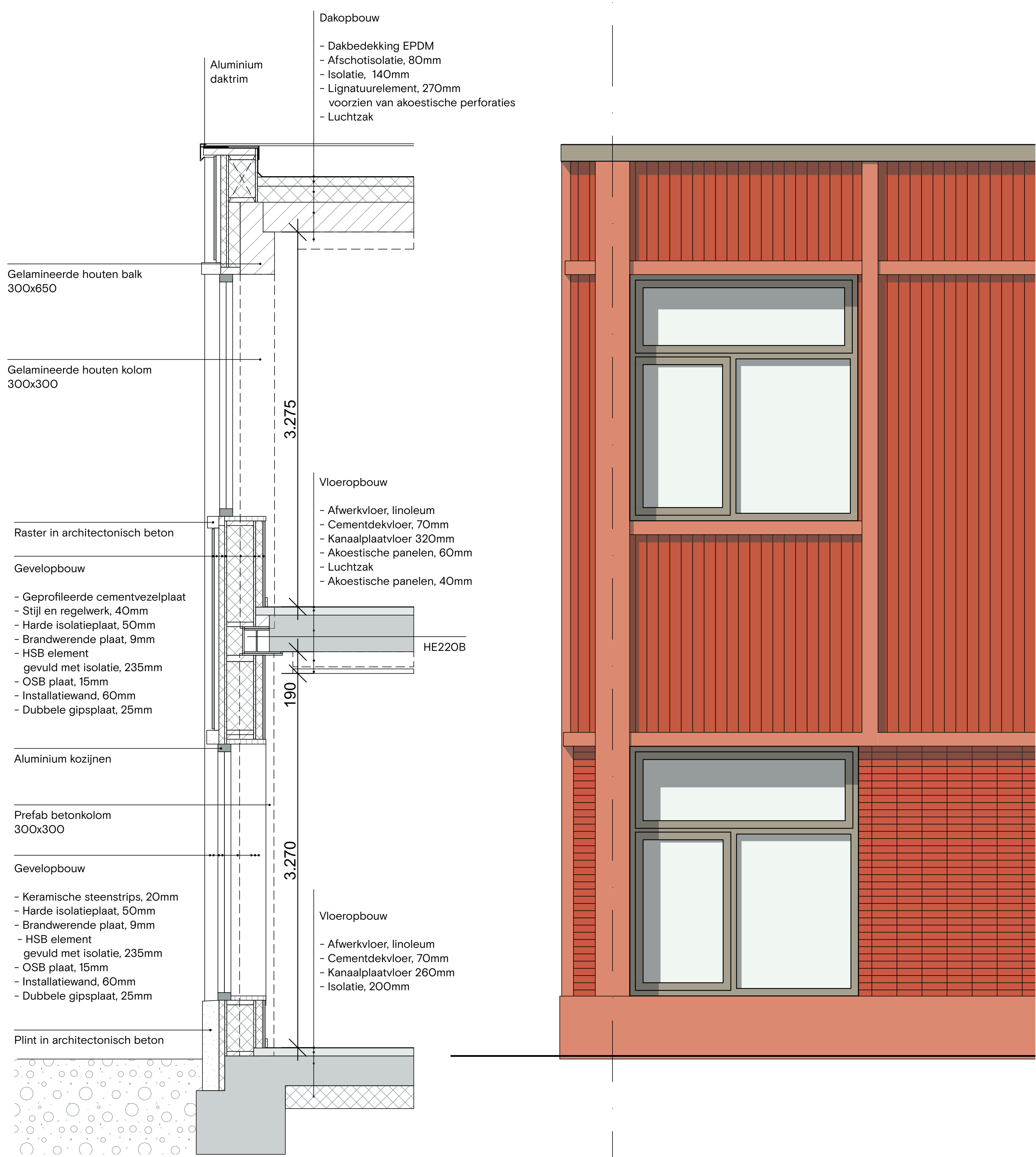
Gevelfragment 1:20
