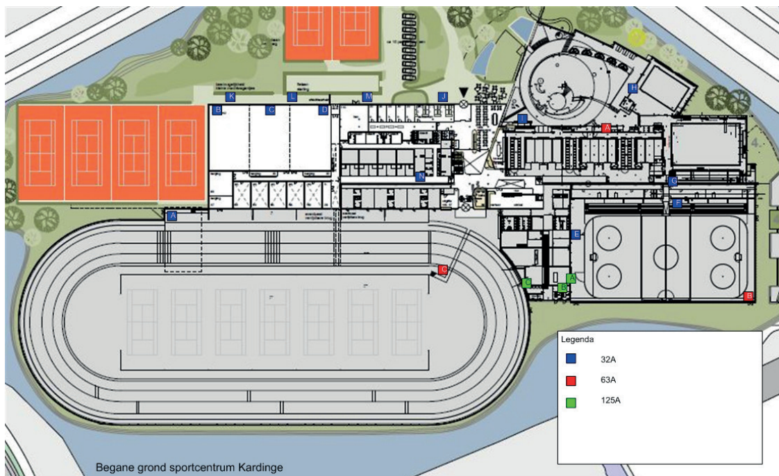
Stroompunten sportcentrum Kardinge begane grond
