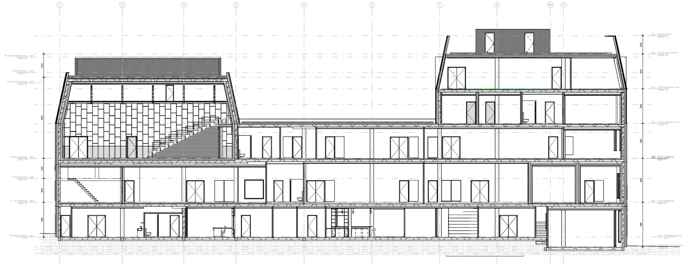
DOORSNEDE A
