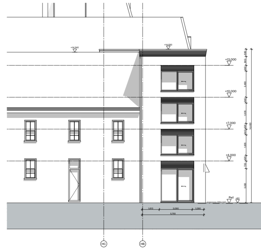
WESTGEVEL
