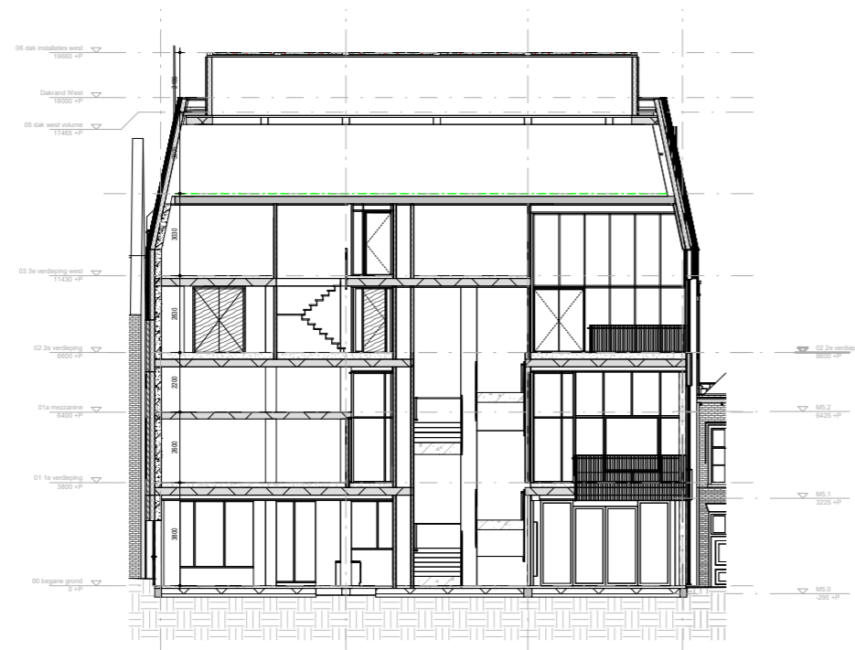
DOORSNEDE B1
