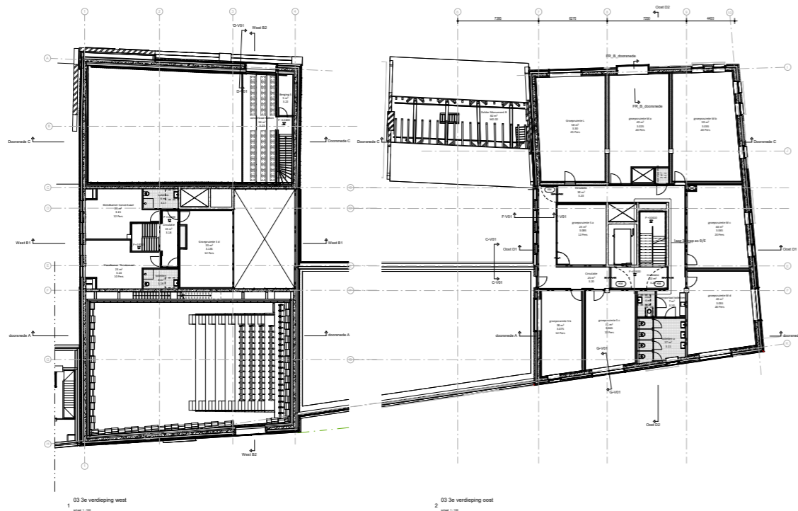
VERDIEPING 3
