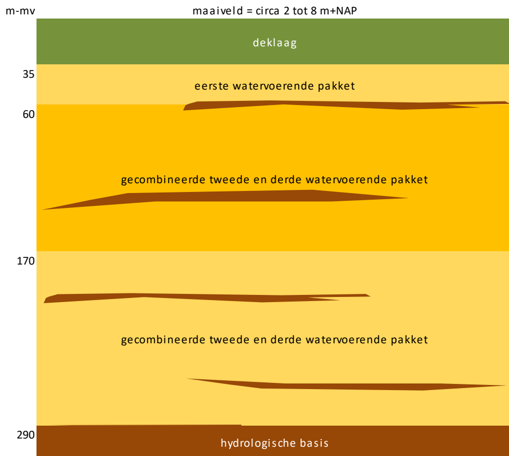
Figuur 3.3 | Schematisatie bodemopbouw
