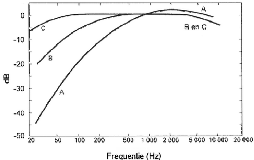
Figuur 4: Verloop van de A, B en C filters per frequentie (wegingsfactor per octaafband)
